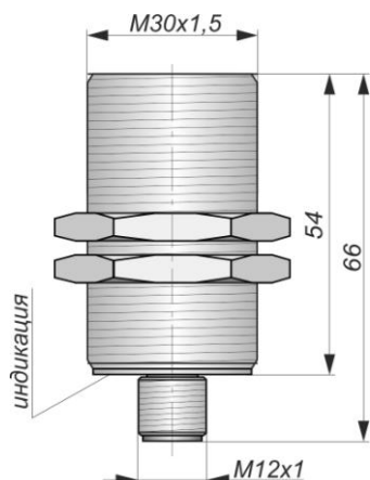
Габаритный чертеж
