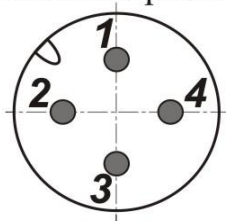
Цоколевка разъема
