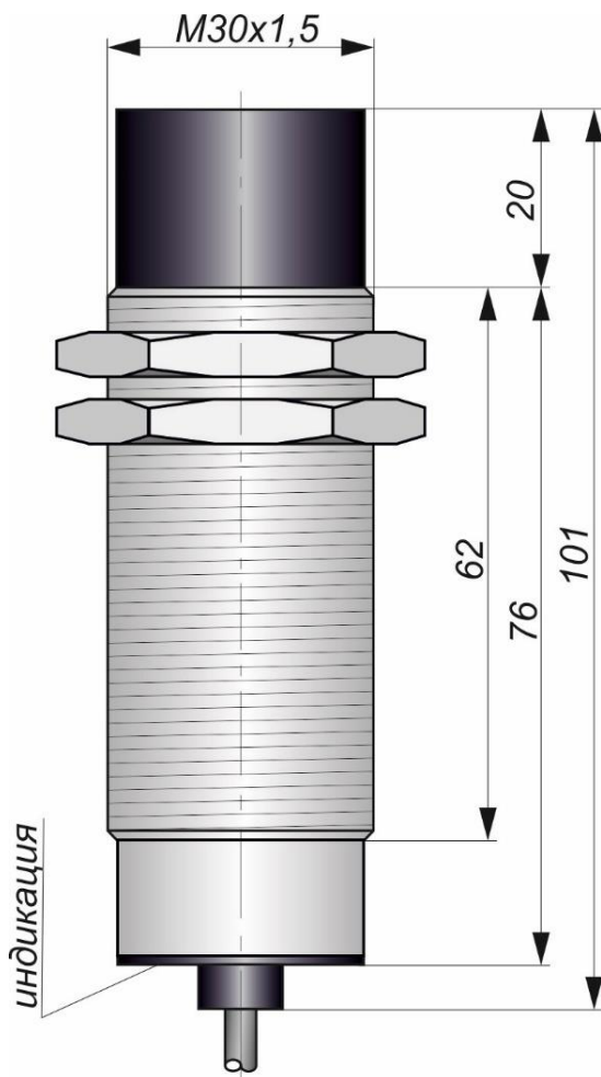
Габаритный чертеж
