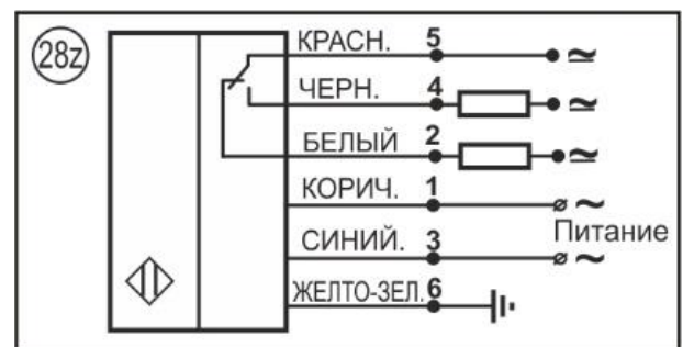
Схема соединения
