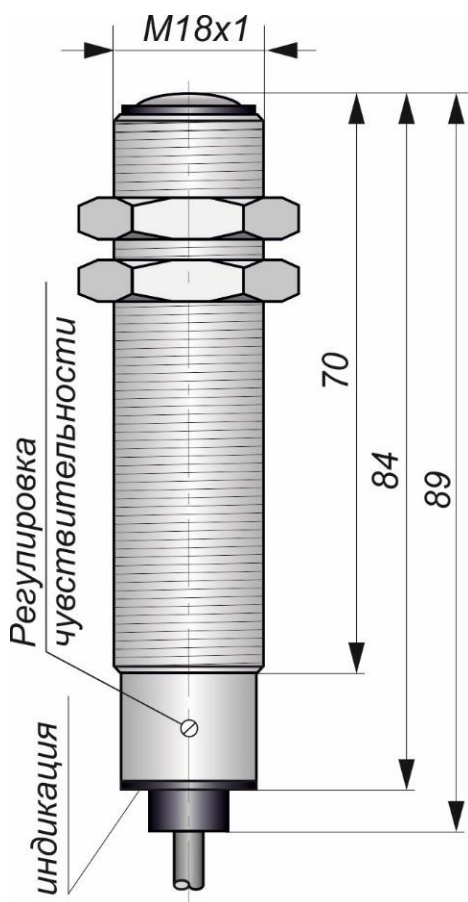
Габаритный чертеж
