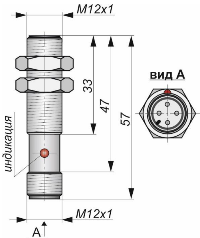
Габаритный чертеж
